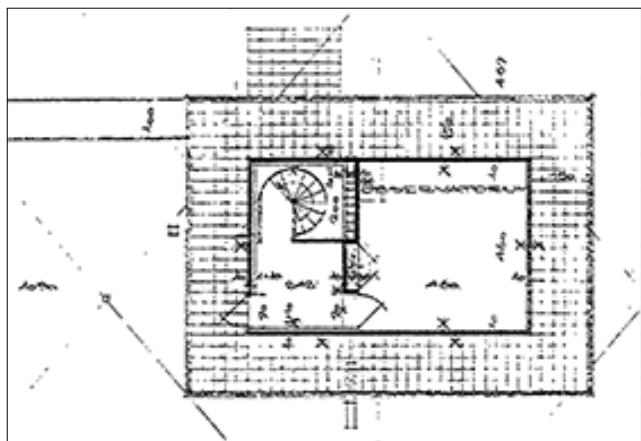
Grundplan over observatoriet med spindeltrappe, forrum med udgang til terrasse og observatorium, hvorpå kuplen blev monteret.
